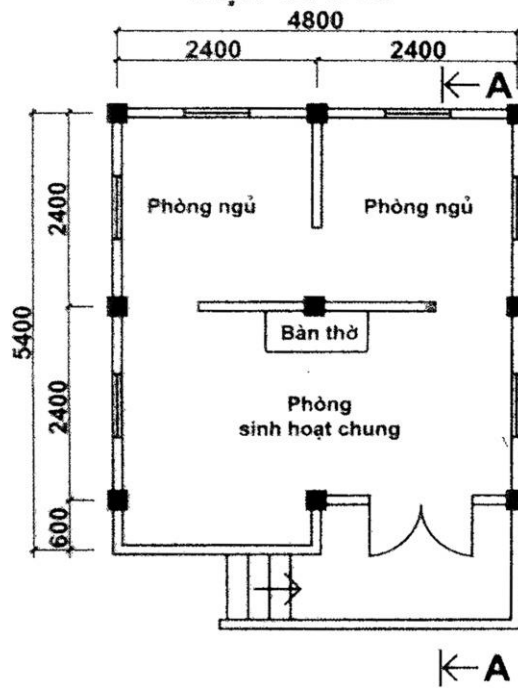
MẶT BẰNG
