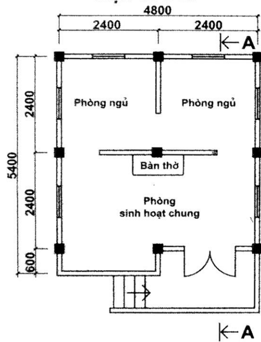
MẶT BẰNG
