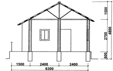
MẶT CẮT A-A
